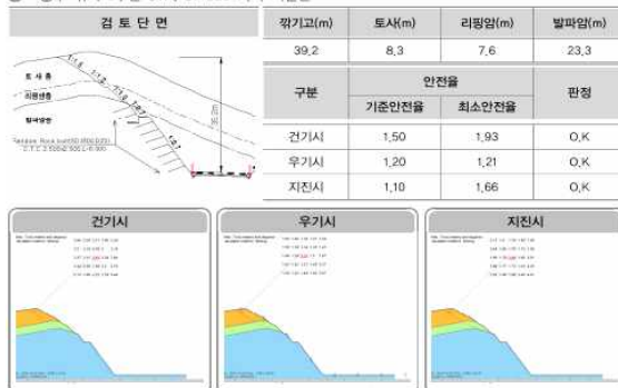
○ 4공구 깎기 6구간 STA. 31+220 좌측 비탈면
