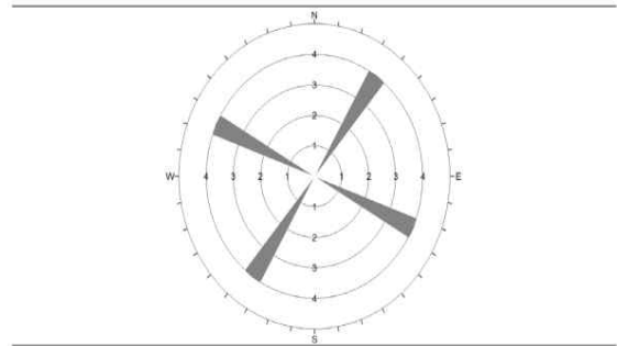
〈그림 16〉 Site-1 절리분포 현황
