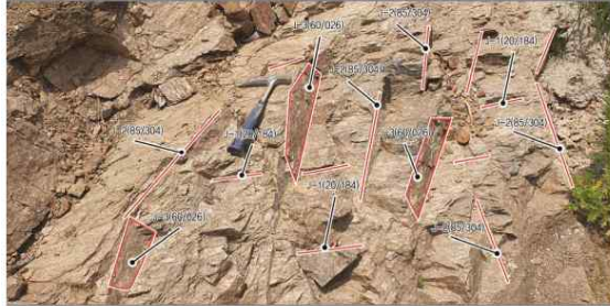
〈그림 14〉 Site-1 비탈면 절리 현황
