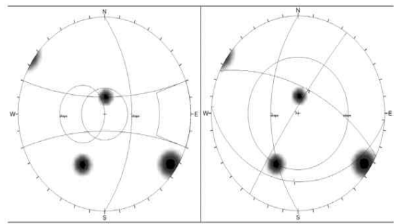
〈그림 15〉 Site-1 편사투영 해석결과
